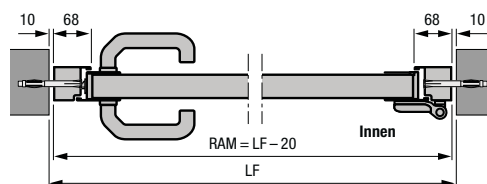
Nebentür mit Alu-Blockzarge Profiltyp 2 Einbau in der Öffnung
