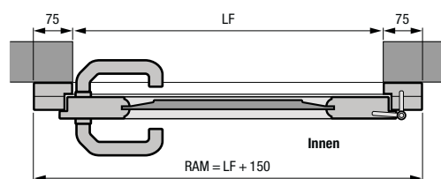
Nebentür aus Massivholz Einbau hinter der Öffnung
