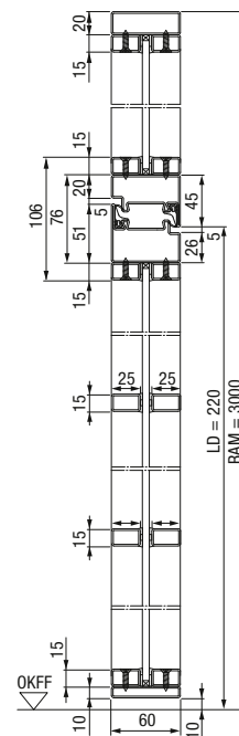
Vertikalschnitt 2-flügelige Stahl-Lofttür mit Seitenteilen und Oberlicht
