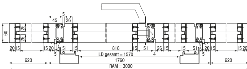
Horizontalschnitt 2-flügelige Stahl-Lofttür mit Seitenteilen und Oberlicht
