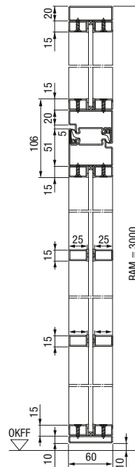
Vertikalschnitt 1-flügelige Stahl-Lofttür mit Seitenteilen und Oberlicht
