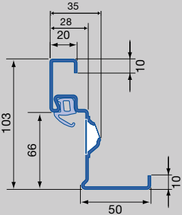
Feuerschutztür EI30, 2-flügelig - Maßanfertigung von - bis / LZ = lichtetes Zargenmaß Türelemente inkl. Zarge in RAL 9002 Grauweiß, inkl. Türschließer TS 4000 und Kunststoff Kurzschild-Drücker D110, schwarz
